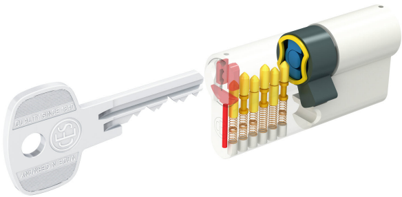
Abb. 6-stiftiges System
